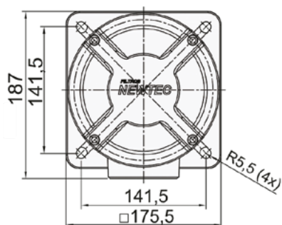
Cabeçote flangeado
